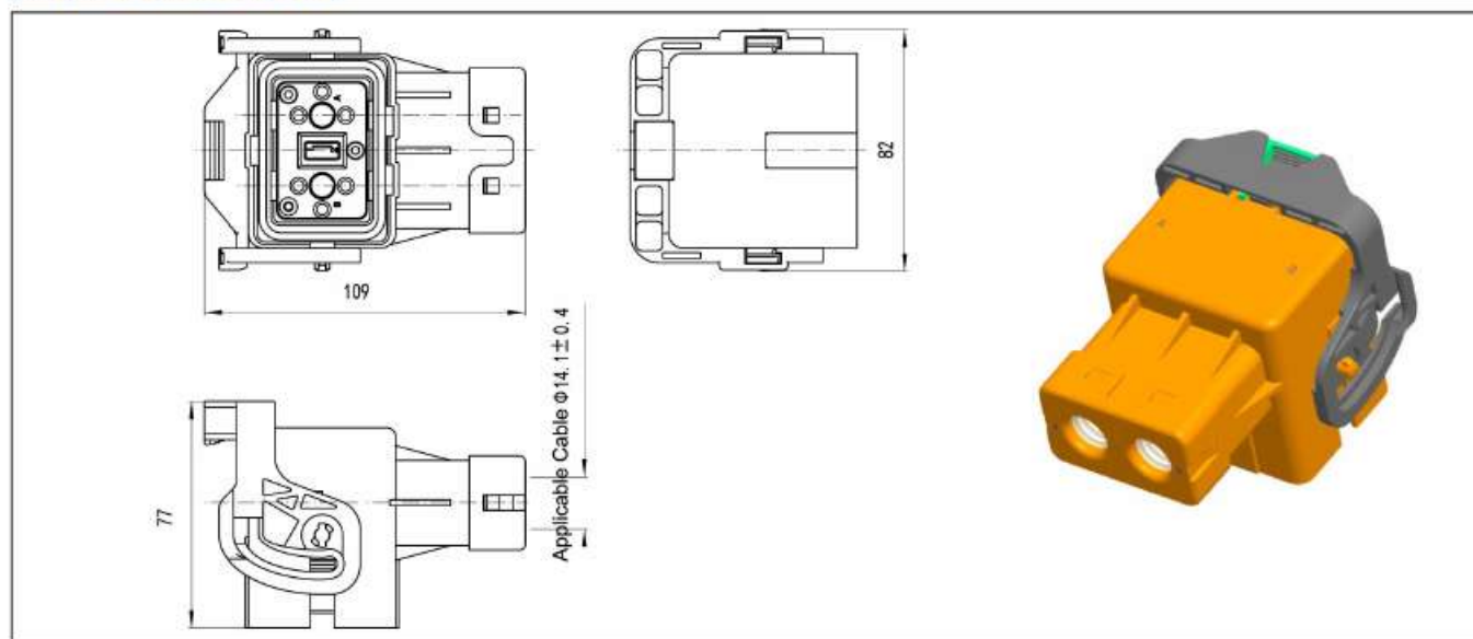
[Plug HVIL-M2S(150A)-90A]
